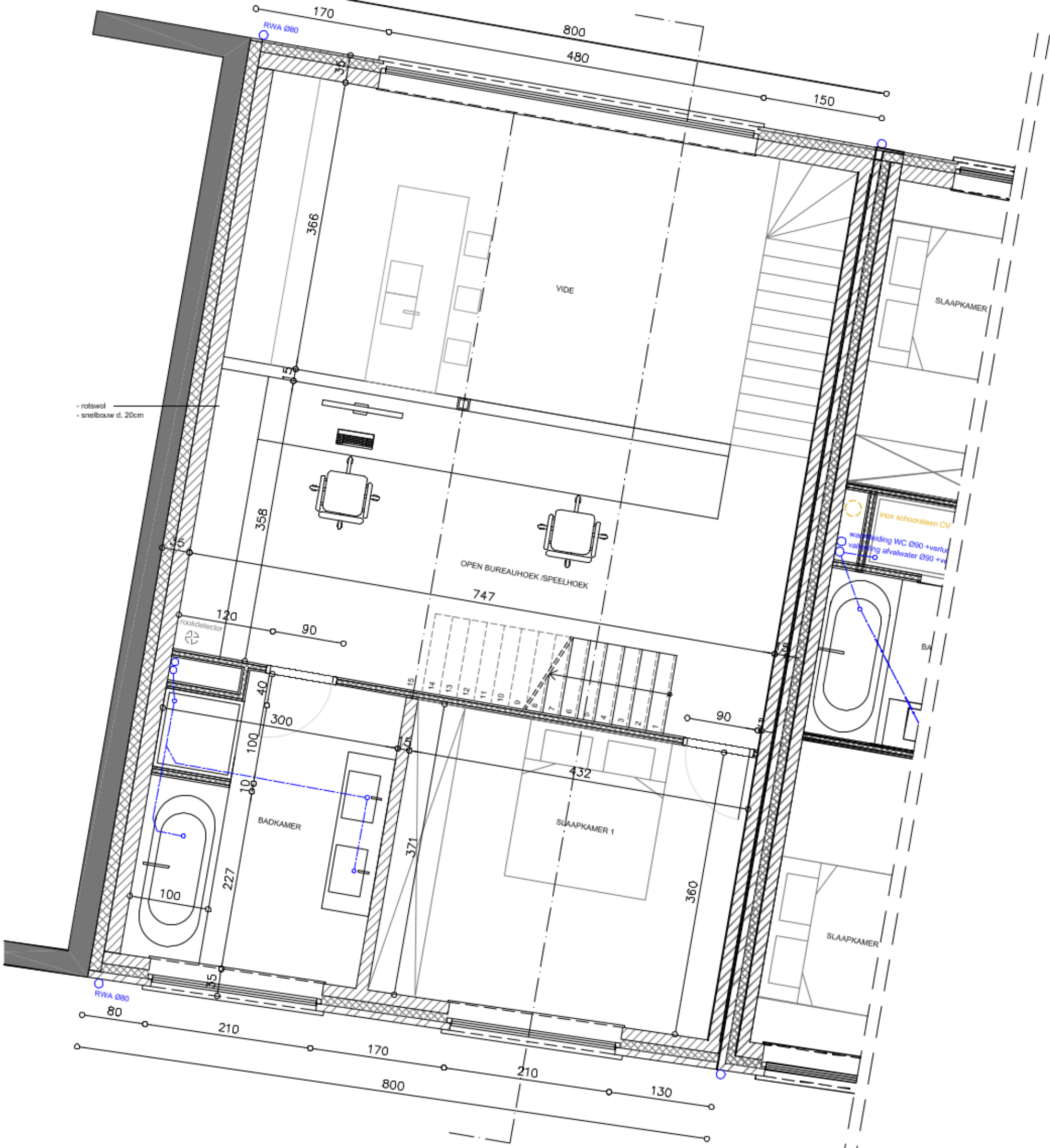
VERDIEPING 01 1/50
