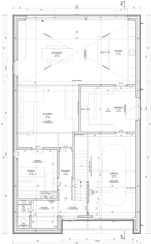
WONING 5 Gelijkvloers: 163,85 m 2
